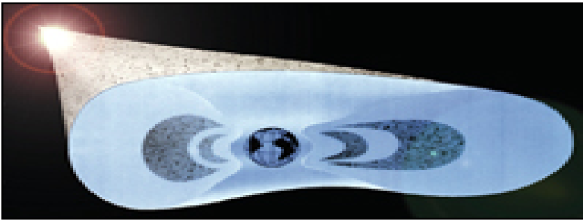
پشتینه کانی تیشکداری زهوی که مرؤف له تیشکی گهردوونی ده پاریزن (Radiation belts)
