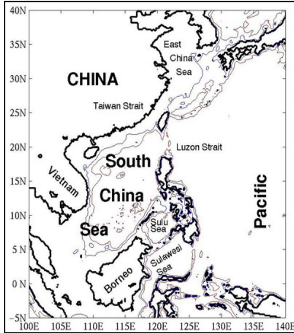
هه‌م وینه‌یه به‌ره‌بستي ناوی نيوآن دهریای باشووری چین و زهریای پاسیفیک روون ده‌کاته‌وه له شوینی به‌یه‌ک گه‌شتنیاندا
