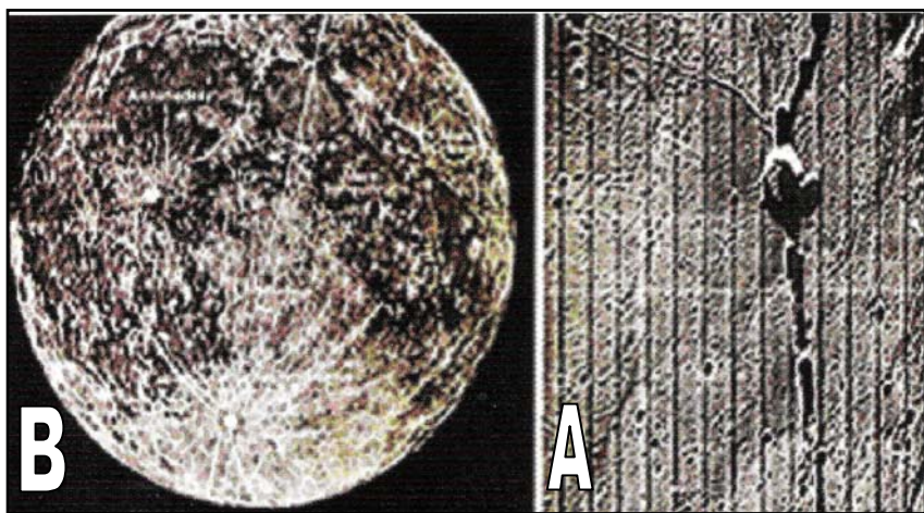
(A) وىنە يەكى راستە قىنەى يەككە لە درزە گەرە و ئاشكراكانى سەر رووى مانگ كە ناسراوھ بە دولتى ھايجىنس (The Hyginus Rille) وىنە يەكى راستە قىنەى مانگ نە كاتى خرىتى تەواو (البدر الكامل) كە درز و قلىشى ناوھراستى رووى مانگ دەرە خات
