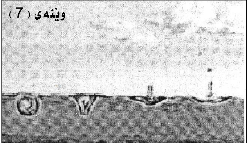
دلۆپه‌ئاوه‌كان ده‌چنه هه‌واوه ، ئه‌مه‌ش يه‌كه‌مين قوناغى دروستبووني هه‌وره‌كانه
