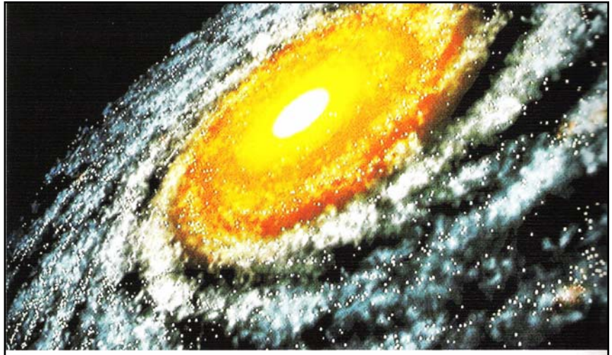
شكل (30) صورة لقرص إحدى المجرات الحلزونية الضخمة
