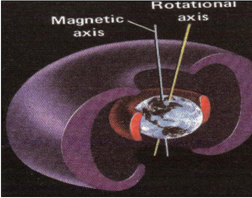
پشتینه کانی تیشکداری زهوی که مرؤف له تیشکی گهردوونی ده پاریزن (Radiation belts)
