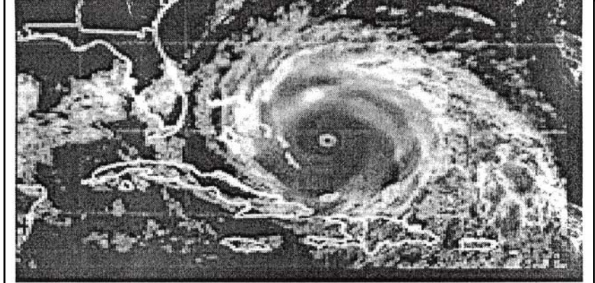
ئه‌م وينه‌يه له‌پرتى مانگه‌ده‌ستكرده‌كانه‌وه گيراوه ، كاربه‌گه‌رى (با) له‌سه‌ر هه‌وره‌كان ده‌رده‌خات كه چۆن وه‌ك ده‌ستيك هه‌ور ئاراسته‌ده‌كات . وينه‌ى (8)
